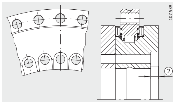
Pour YRTS325 : ② Lamages des vis dégagés 5)
