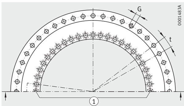
Schéma de perçage ① Deux vis d'assemblage
