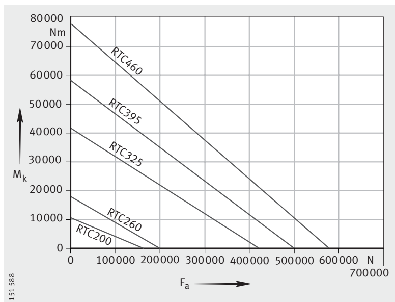
Figure 9 Diagramme des charges statiques limites pour RTC200 à RTC460
