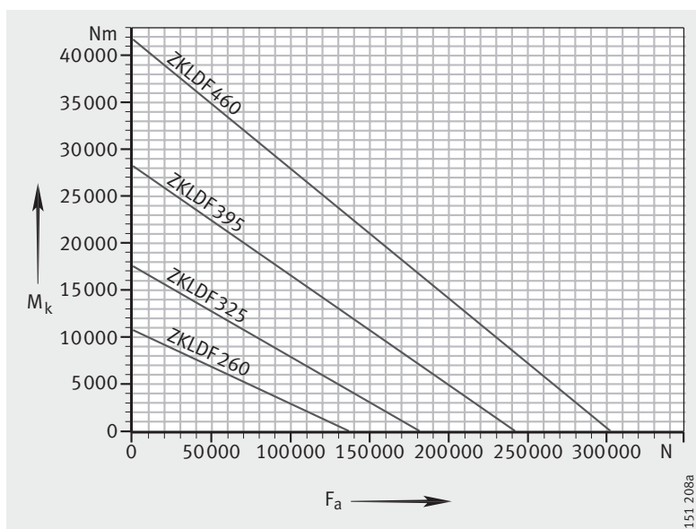
Figure 11 Diagramme des charges statiques limites pour ZKLDF260 à ZKLDF460
