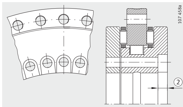
Pour YRT325 : ② Lamages des vis dégagés 5)
